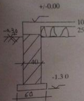
Coupe 1-1
