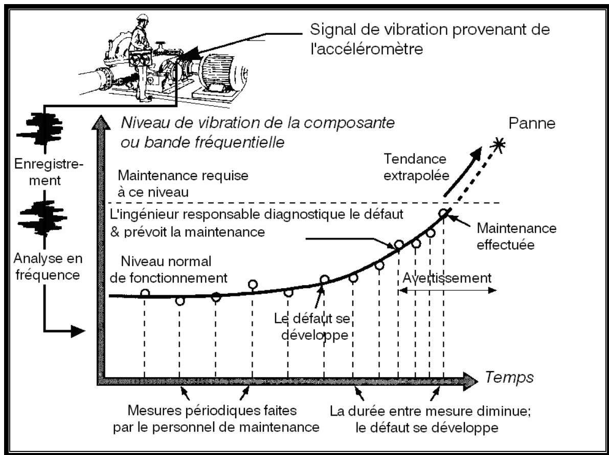
Fig. 6a. Principe de la surveillance vibratoire d'une machine
