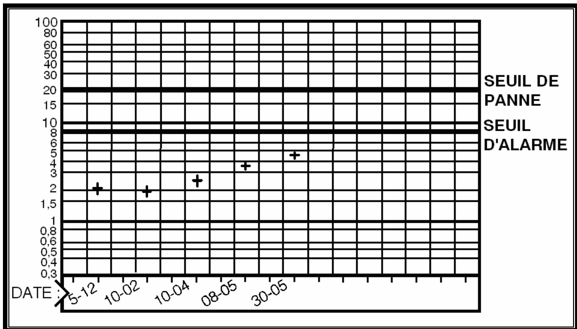
Fig. 6c. Enregistrement des valeurs mesurées
