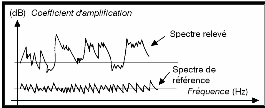
Fig. 6b. Comparaison entre les deux spectres de vibration
