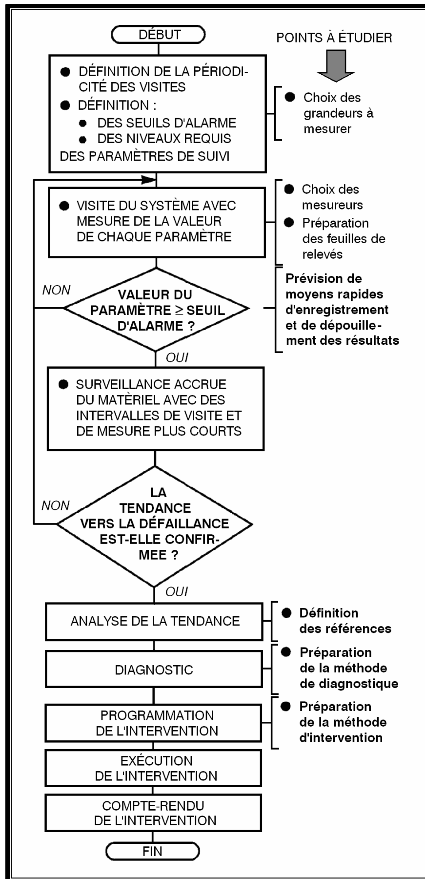
Fig. 5a. Organisation du l'entretien préventif prévisionnel et points à étudier pour sa mise en oeuvre
