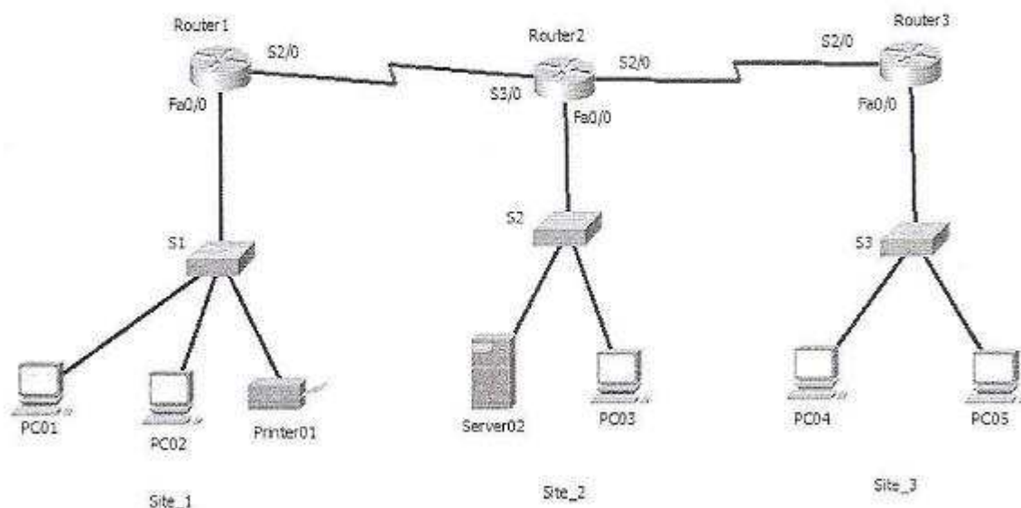
Schéma de l'architecture réseau
